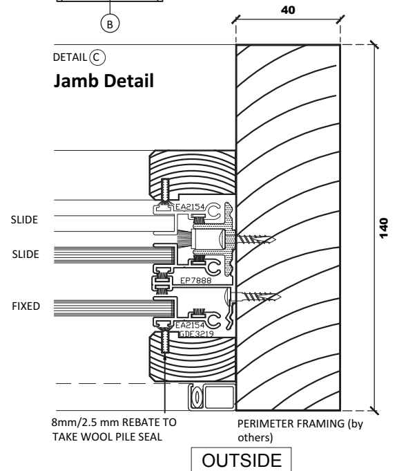
DETAIL (D) Jamb Detail
