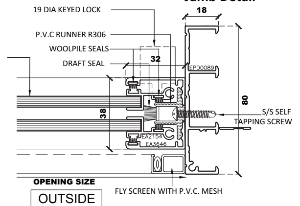
Jamb Detail
