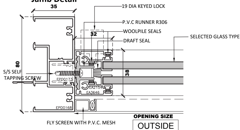
Jamb Detail
