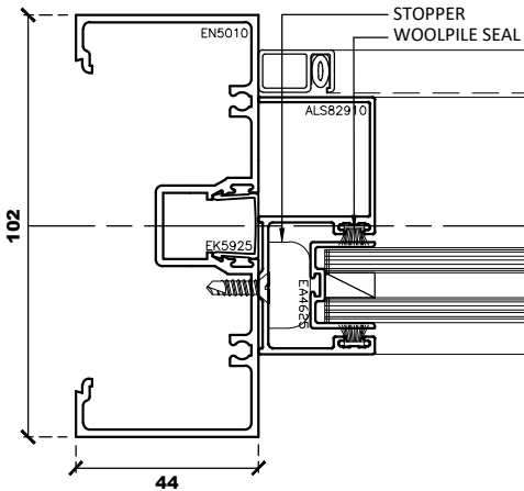
Jamb Detail
