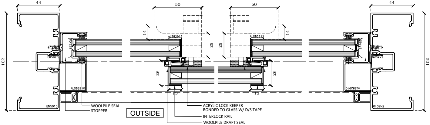
Jamb Detail
