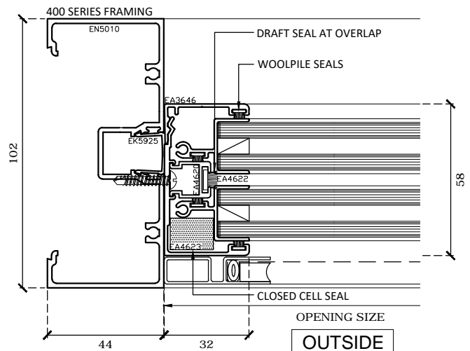
C Jamb Detail
